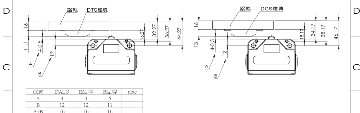
LS-D2/D3限動開關與鋁軌碰塊安裝說明
